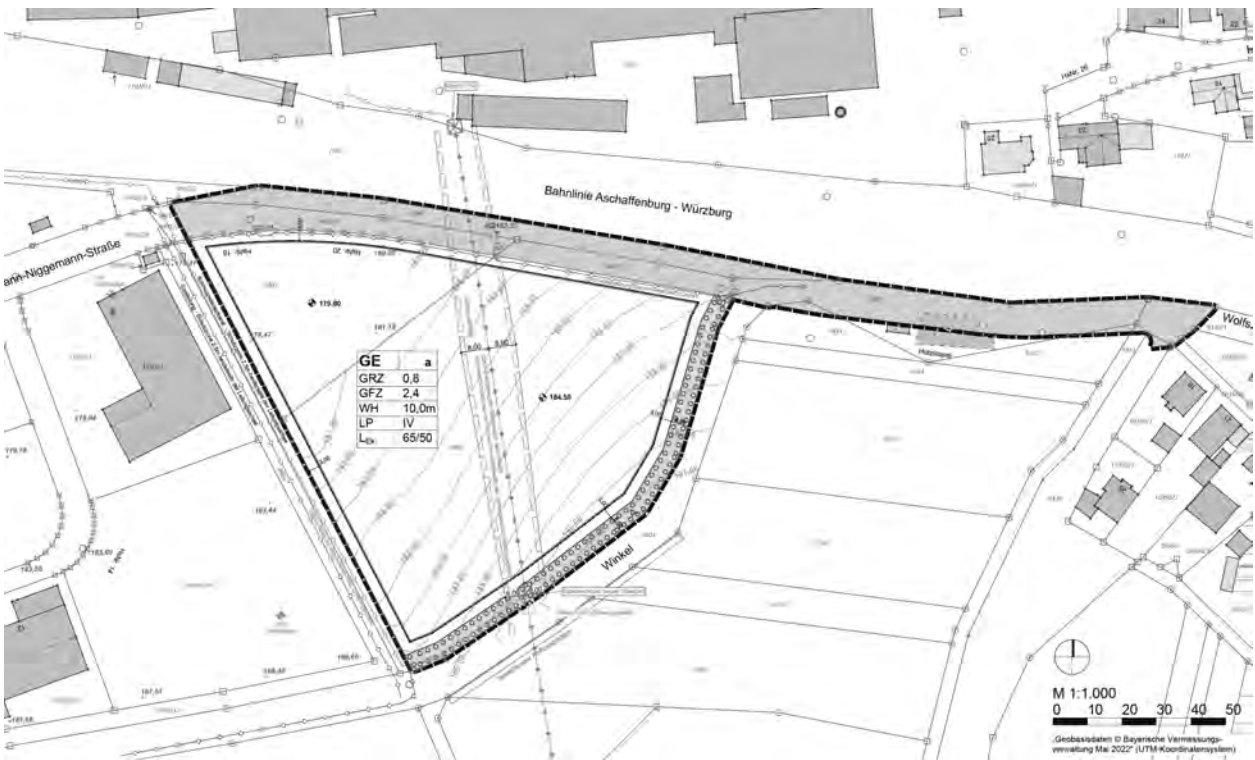
Entwurf des Bebauungs- und Grünordnungsplans
