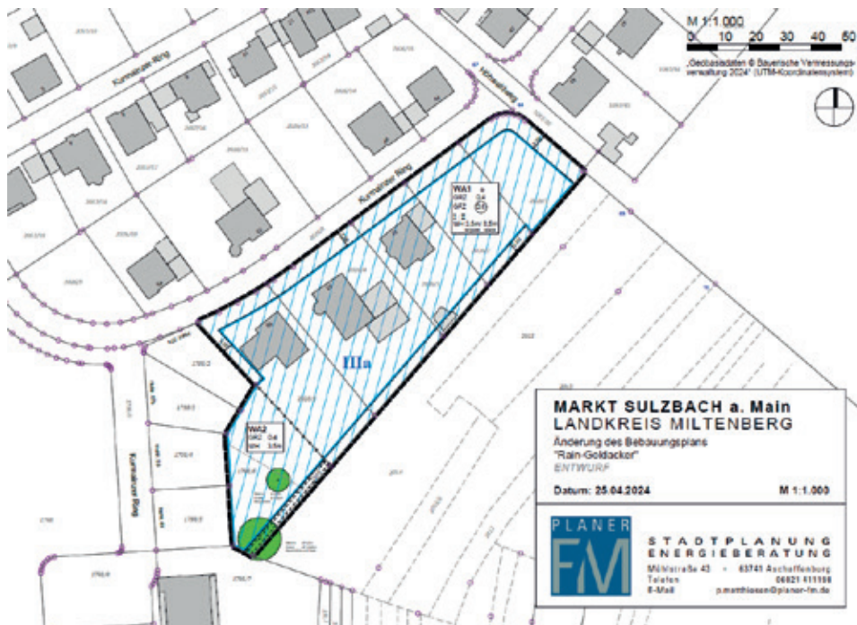
Bebauungsplanänderungsentwurf (unmaßstäblich)
